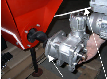
Afmontering af snegl og gear. Ved afmontering af motor kontroller da at ledning bliver monteret korrekt
