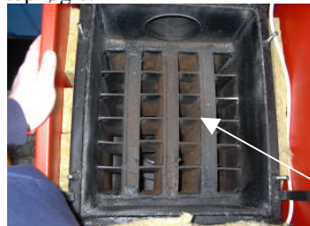
Rens samtlige røg kanaler med den medfølgende børste.
