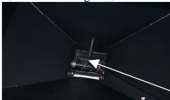
Bund af magasin snegl og ind løbs rør fra brandslukning
