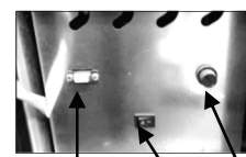
RS 232 SIKKERHEDS TERMOSTAT ON/OFF AFBRYDER
